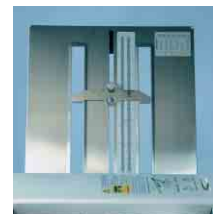
Falzartenschnelleinstellung und -feinjustierung mit selbsterklärender Skala
